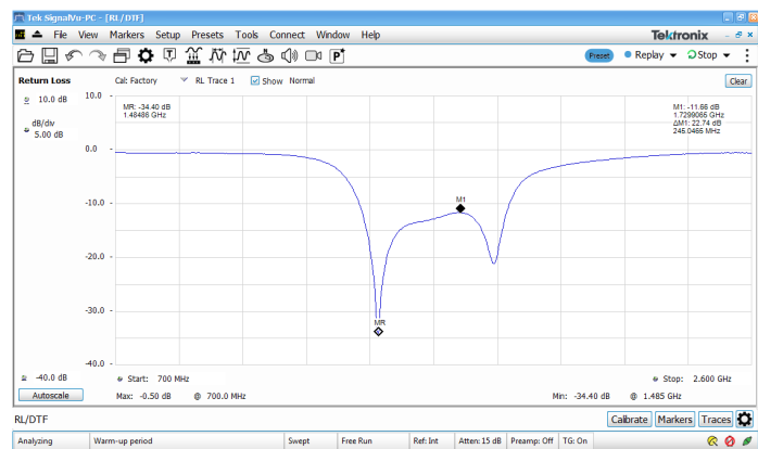
从 700 MHz 至 2.6 GHz 测得的通带滤波器的回波损耗。标记被放在 1.48 GHz (-34.4 dB 回波损耗) 和 1.73 GHz (-11.68 dB 回波损耗) 处，指明滤波器通带中的最佳匹配和最差匹配。
