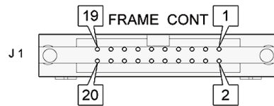
J1 连接器
