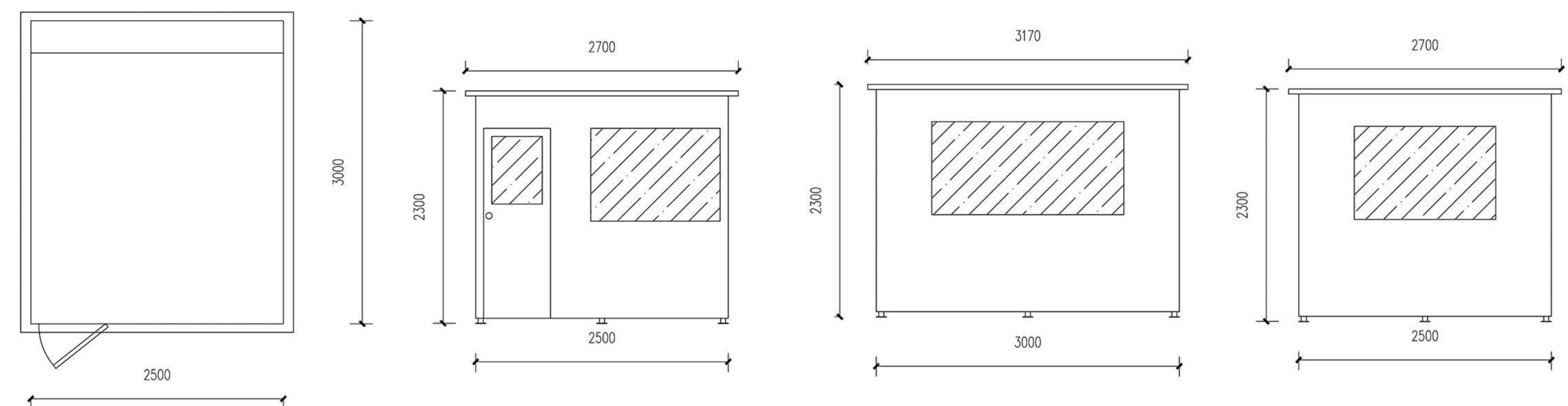
-План этажа-
