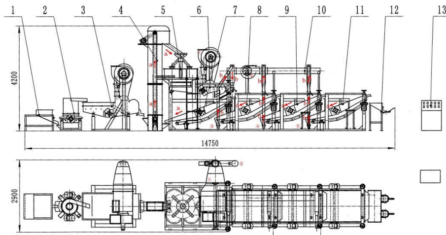
ОБОРУДОВАНИЕ ДЛЯ ОЧИСТКИ, ШЕЛУШЕНИЯ И СЕПАРАЦИИ СЕМЯН ПОДСОЛНЕЧНИКА TFKN-1500
