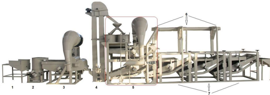
Оборудование для шелушения семечки подсолнечника TFKN-1500-горизонтальный тип
