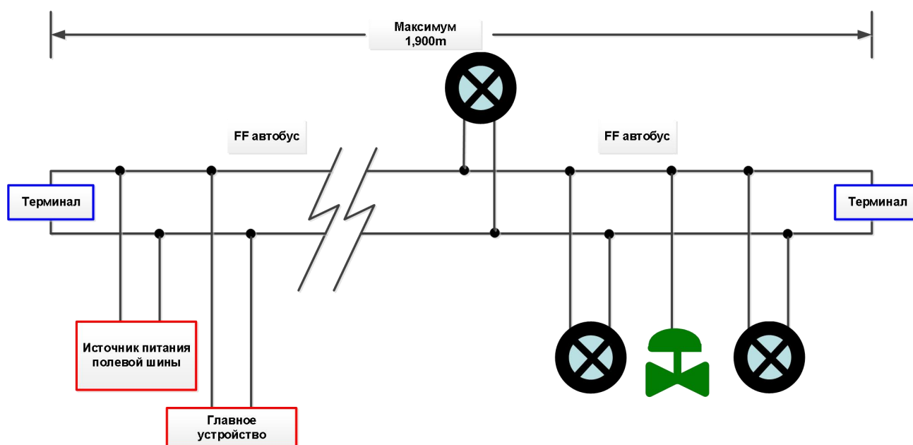
Рисунок 6 . 1 Топология сети FF
