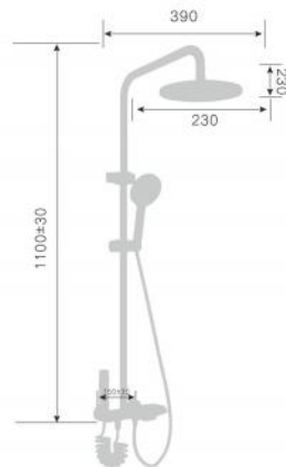
250003Q-T Тропический душ со смесителем Single level rain shower mixer Количество упаковок в коробку:6 Packing count:6
