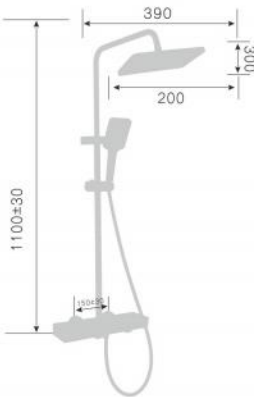
250024D-T Тропический душ со смесителем Single level rain shower mixer Количество упаковок в коробку: 6 Packing count: 6
