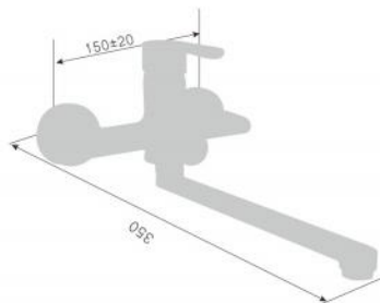
220049D-T Смеситель для ванны с переключателем в корпусе Single lever wall-mounted kitchen shower mixer Количество упаковок в коробку: 10 Packing count: 10
