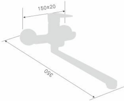
220028D-X Смеситель для ванны с переключателем в корпусе Single lever wall-mounted kitchen shower mixer Количество упаковок в коробку: 10 Packing count: 10
