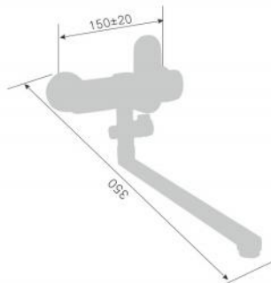
220038D-T Смеситель для ванны с переключателем в корпусе Single lever wall-mounted kitchen shower mixer Количество упаковок в коробку: 10 Packing count: 10
