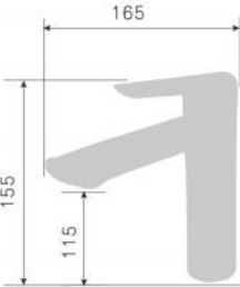
200111D-T 200111Q-T смеситель для раковины Single lever basin mixer Количество упаковок в коробку: 18 Packing count: 18
