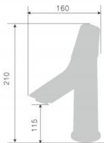
200139D-X 200139Q-X 200139H-X смеситель для раковины Single lever basin mixer Количество упаковок в коробку: 18 Packing count: 18
