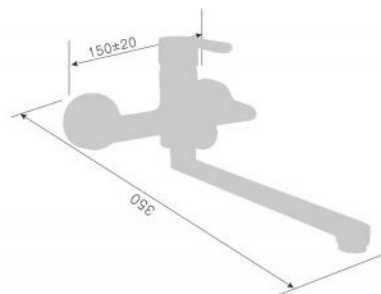
220002D-T Смеситель для ванны с переключателем в корпусе Single lever wall-mounted kitchen shower mixer Количество упаковок в коробку: 110 Packing count: 10
