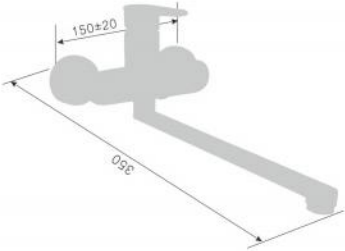
220001D-T Смеситель для ванны с переключателем в корпусе Single lever wall-mounted kitchen shower mixer Количество упаковок в коробку: 10 Packing count: 10
