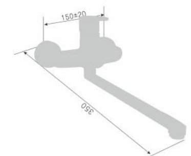
220029D-T Смеситель для ванны с переключателем в корпусе Single lever wall-mounted kitchen shower mixer Количество упаковок в коробку: 10 Packing count: 10
