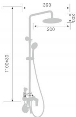
250033D-T 250033H-T Тропический душ со смесителем Single level rain shower mixer Количество упаковок в коробку: 6 Packing count: 6
