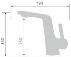
200146D-X 200146Q-X 200146J-X смеситель для раковины Single lever basin mixer Количество упаковок в коробку: 18 Packing count: 18
