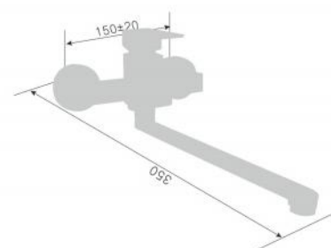
220013D-T Смеситель для ванны с переключателем в корпусе Single lever wall-mounted kitchen shower mixer Количество упаковок в коробку: 10 Packing count: 10
