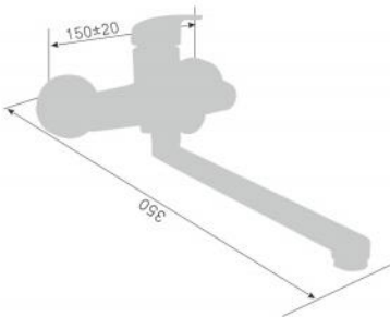
220019Q-S Смеситель для ванны с переключателем в корпусе Single lever wall-mounted kitchen shower mixer Количество упаковок в коробку: 10 Packing count: 10
