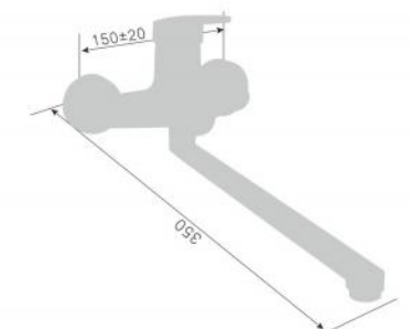
220045D-X Смеситель для ванны с переключателем в корпусе Single lever wall-mounted kitchen shower mixer Количество упаковок в коробку: 10 Packing count: 10
