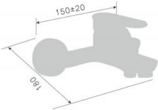
240001D-T Смеситель для ванны с переключателем в корпусе Single lever bath shower mixer Количество упаковок в коробку: 18 Packing count: 18
