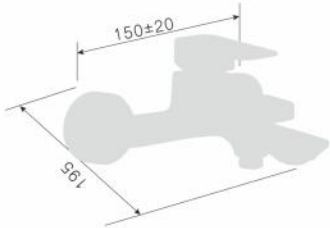
240007D-X Смеситель для ванны с переключателем в корпусе Single lever bath shower mixer Количество упаковок в коробку: 18 Packing count: 18
