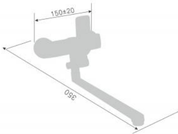
220036D-T Смеситель для ванны с переключателем в корпусе Single lever wall-mounted kitchen shower mixer Количество упаковок в коробку: 10 Packing count: 10
