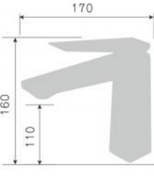
200112D-T 200112Q-T смеситель для раковины Single lever basin mixer Количество упаковок в коробку: 18 Packing count: 18
