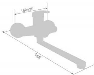
220044D-X Смеситель для ванны с переключателем в корпусе Single lever wall-mounted kitchen shower mixer Количество упаковок в коробку: 10 Packing count: 10
