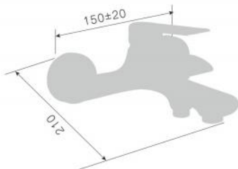
240004D-T Смеситель для ванны с пе реключателем в корпусе Single lever bath shower mixer Количество упаковок в коробку: 18 Packing count: 18
