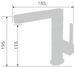
200016D-X 200016Q-X смеситель для раковины Single lever basin mixer Количество упаковок в коробку: 18 Packing count: 18
