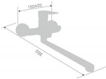
220035D-T Смеситель для ванны с переключателем в корпусе Single lever wall-mounted kitchen shower mixer Количество упаковок в коробку: 10 Packing count: 10
