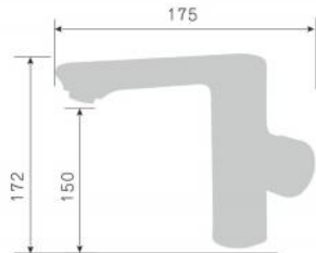
200081D-X 200081Q-X 200081B-X смеситель для раковины Single lever basin mixer Количество упаковок в коробку: 18 Packing count: 18
