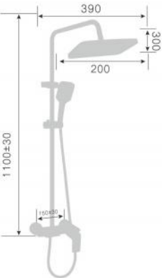
250036D-T Тропический душ со смесителем Single level rain shower mixer Количество упаковок в коробку: 6 Packing count: 6
