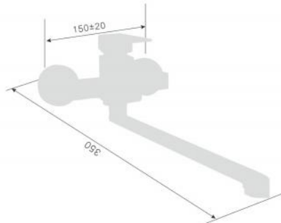
220027D-X Смеситель для ванны с переключателем в корпусе Single lever wall-mounted kitchen shower mixer Количество упаковок в коробку: 10 Packing count: 10
