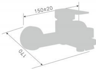
240027D-X Смеситель для ванны с переключателем в корпусе Single lever bath shower mixer Количество упаковок в коробку: 18 Packing count: 18
