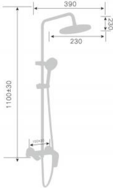
250040D-T 250040Q-T Тропический душ со смесителем Single level rain shower mixer Количество упаковок в коробку: 6 Packing count: 6
