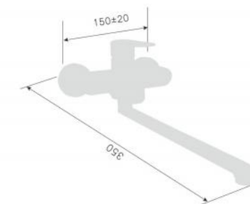
220005D-X Смеситель для ванны с переключателем в корпусе Single lever wall-mounted kitchen shower mixer Количество упаковок в коробку: 10 Packing count: 10
