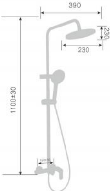
250013D-T 250013Q-T Тропический душ со смесителем Single level rain shower mixer Количество упаковок в коробку: 6 Packing count: 6
