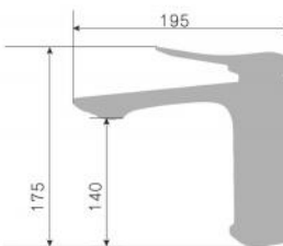
200073D-X 200073Q-X 200073H-X смеситель для раковины Single lever basin mixer Количество упаковок в коробку: 18 Packing count: 18
