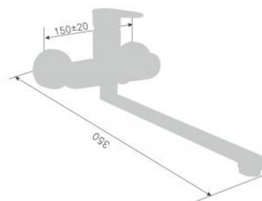
220017D-X Смеситель для ванны с переключателем в корпусе Single lever wall-mounted kitchen shower mixer Количество упаковок в коробку: 10 Packing count: 10
