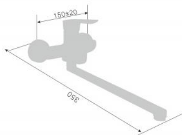
220042D-T Смеситель для ванны с переключателем в корпусе Single lever wall-mounted kitchen shower mixer Количество упаковок в коробку: 10 Packing count: 10
