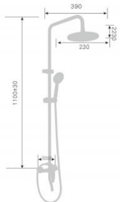
250049D-T Тропический душ со смесителем Single level rain shower mixer Количество упаковок в коробку: 6 Packing count:6
