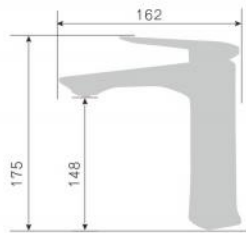
200079H-X смеситель для раковины Single lever basin mixer Количество упаковок в коробку: 18 Packing count: 18
