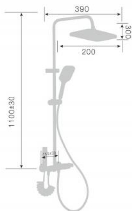
250020D-T 250020Q-T Тропический душ со смесителем Single level rain shower mixer Количество упаковок в коробку: 6 Packing count: 6
