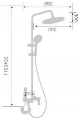
250027D-T Тропический душ со смесителем Single level rain shower mixer Количество упаковок в коробку: 6 Packing count: 6
