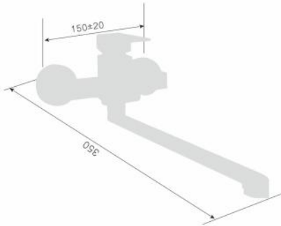
220007D-X Смеситель для ванны с переключателем в корпусе Single lever wall-mounted kitchen shower mixer Количество упаковок в коробку: 10 Packing count: 10
