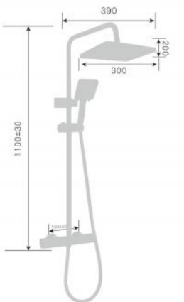
250054D-T Тропический душ со смесителем Single level rain shower mixer Количество упаковок в коробку:6 Packing count:6
