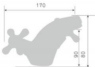
270004D-T смеситель для раковины Single lever basin mixer Количество упаковок в коробку: 18 Packing count: 18
