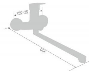
220015D-X Смеситель для ванны с переключателем в корпусе Single lever wall-mounted kitchen shower mixer Количество упаковок в коробку: 10 Packing count: 10
