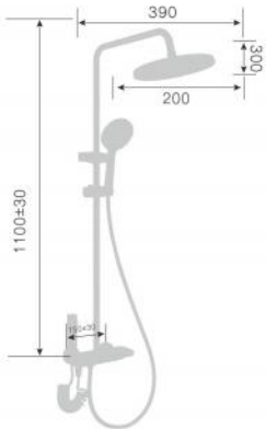
250028D-T Тропический душ со смесителем Single level rain shower mixer Количество упаковок в коробку: 6 Packing count: 6
