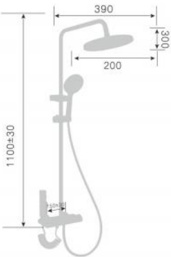
250022D-T Тропический душ со смесителем Single level rain shower mixer Количество упаковок в коробку: 6 Packing count: 6
