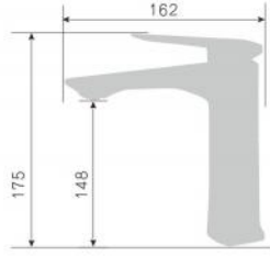
200079J-X смеситель для раковины Single lever basin mixer Количество упаковок в коробку: 18 Packing count: 18
