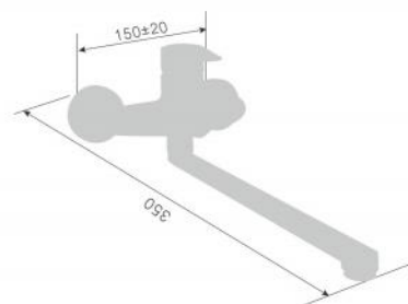
220037Q-T Смеситель для ванны с переключателем в корпусе Single lever wall-mounted kitchen shower mixer Количество упаковок в коробку: 10 Packing count: 10
