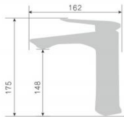
200079D-X смеситель для раковины Single lever basin mixer Количество упаковок в коробку: 18 Packing count: 18
