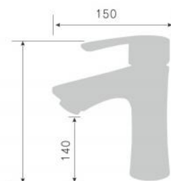
200025D-T смеситель для раковины Single lever basin mixer Количество упаковок в коробку: 18 Packing count: 18
