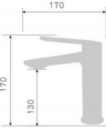
200110D-T 200110Q-T смеситель для раковины Single lever basin mixer Количество упаковок в коробку: 18 Packing count: 18
