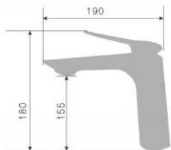
200072D-X 200072Q-X 200072J-X смеситель для раковины Single lever basin mixer Количество упаковок в коробку: 18 Packing count: 18
