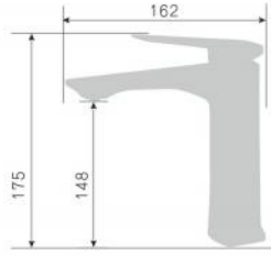
200079Q-X смеситель для раковины Single lever basin mixer Количество упаковок в коробку: 18 Packing count: 18
