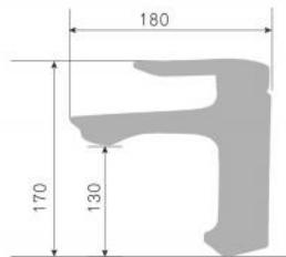
200039D-X 200039Q-X 200039H-X смеситель для раковины Single lever basin mixer Количество упаковок в коробку: 18 Packing count: 18
