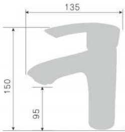
200109D-T 200109Q-T смеситель для раковины Single lever basin mixer Количество упаковок в коробку: 18 Packing count: 18
