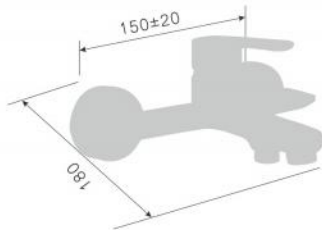
240002D-T Смеситель для ванны с переключателем в корпусе Single lever bath shower mixer Количество упаковок в коробку: 18 Packing count: 18
