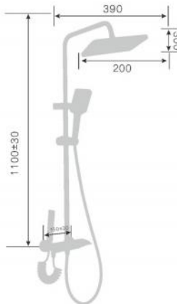
250030D-T Тропический душ со смесителем Single level rain shower mixer Количество упаковок в коробку: 10 Packing count: 10
