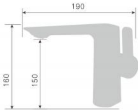
200080D-X 200080Q-X 200080J-X смеситель для раковины Single lever basin mixer Количество упаковок в коробку: 18 Packing count: 18
