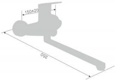
220053D-T Смеситель для ванны с переключателем в корпусе Single lever wall-mounted kitchen shower mixer Количество упаковок в коробку: 10 Packing count: 10
