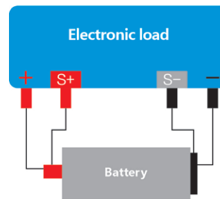
▲ Discharge Wiring
