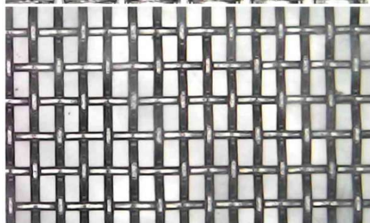
API RP 13C - расшифровка Номеров ситовых панелей
