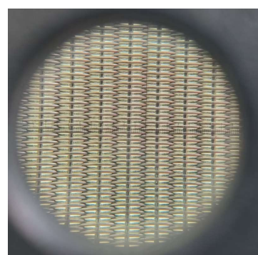
✓ П40-12X18Н10Т ГОСТ 3187-76
